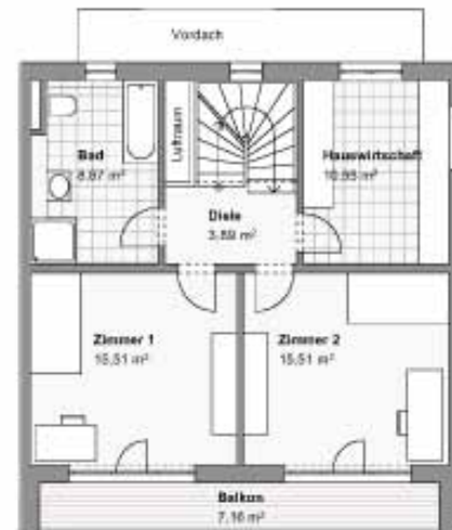
Grundriss 1.OG
