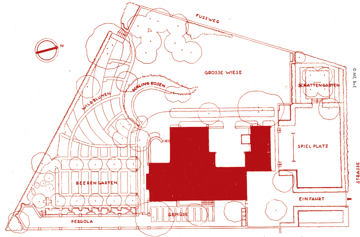
Haus Elsaesser, Lageplan
