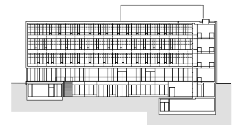
Biologicum Querschnitt
