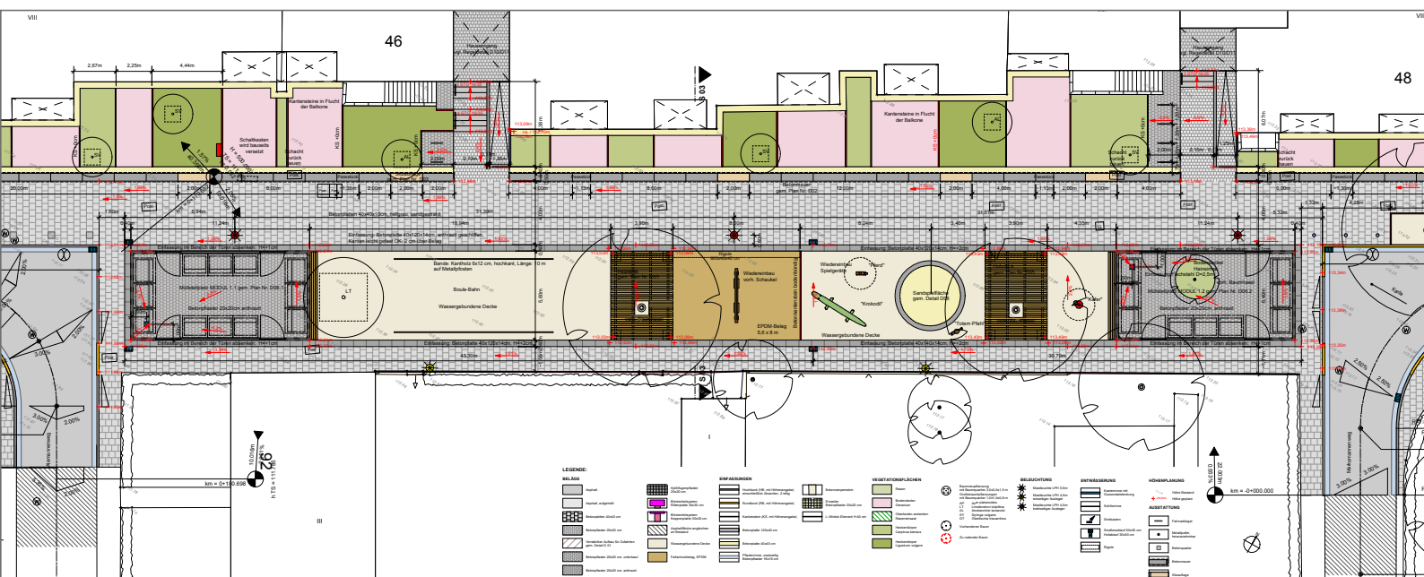
Aufweitung West, Ausführungsplanung: Landschaftsarchitekten Mann (Fulda)
