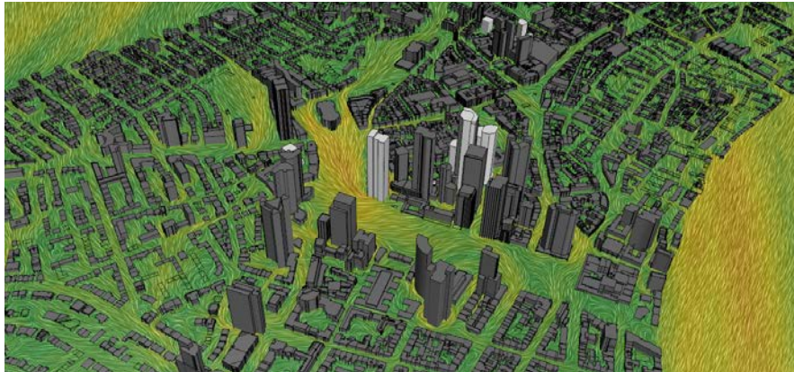
Detailansicht Bankenviertel 20 m über Grund
