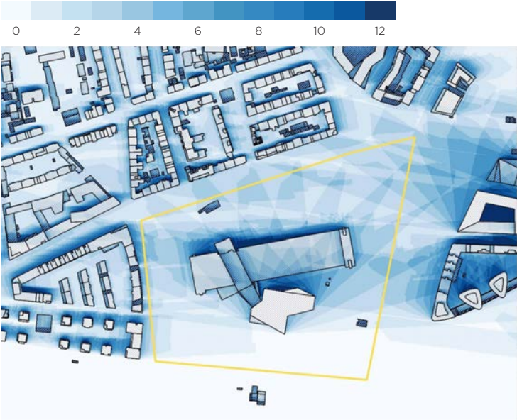
21. SEPTEMBER 2023 (MAX. 12 STUNDEN) ANZAHL DER STUNDEN MIT SCHATTEN
