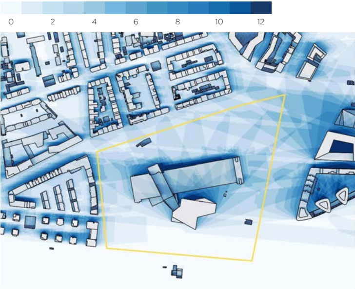
21. MÄRZ 2023 (MAX. 12 STUNDEN) ANZAHL DER STUNDEN MIT SCHATTEN
