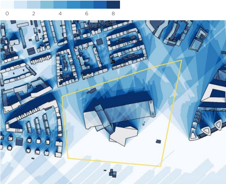
21. DEZEMBER 2023 (MAX. 8 STUNDEN) ANZAHL DER STUNDEN MIT SCHATTEN
