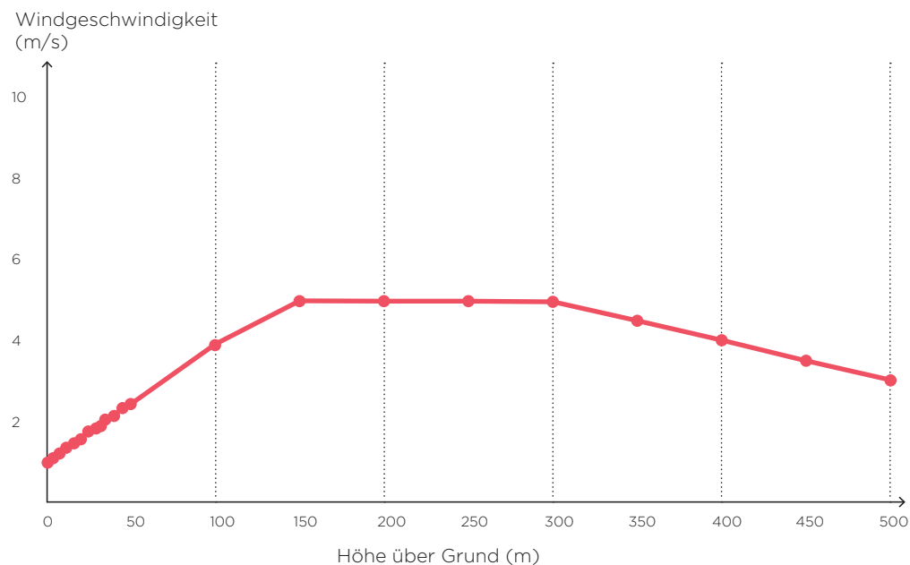
Vertikales Windprofil für den einströmenden Wetterauwind am östlichen und nördlichen Rand der Computerdomäne
