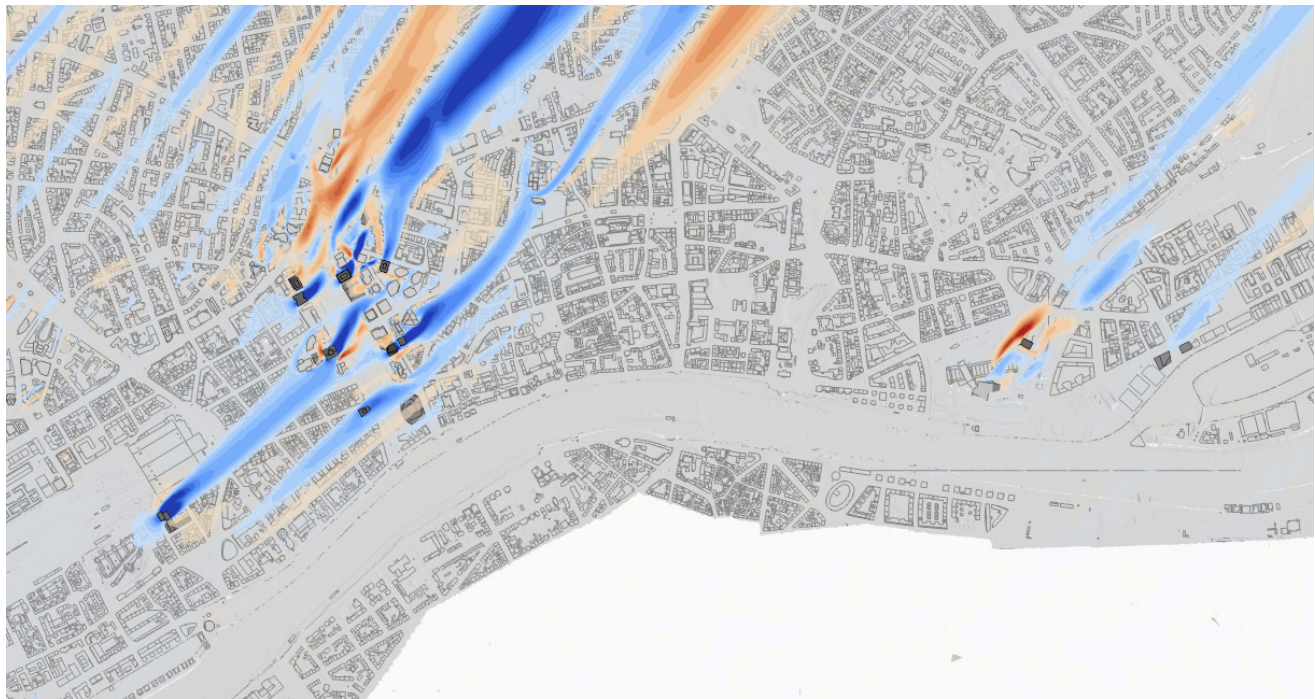
100 m über Grund
