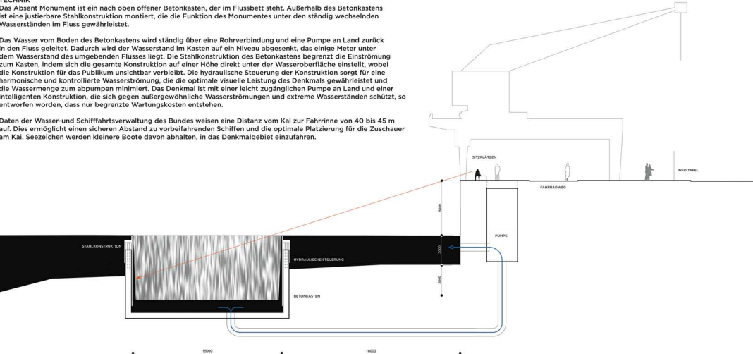
SCHNITT 1100
